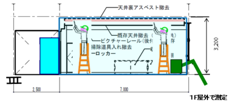
作業場所断面図
