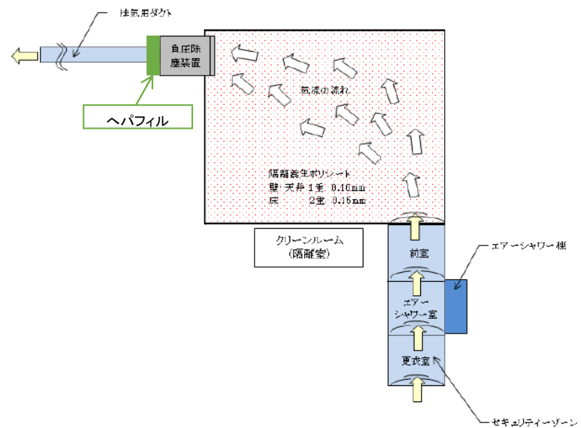
セキュリティーゾーン、クリーンルーム配置例 (平面図)
