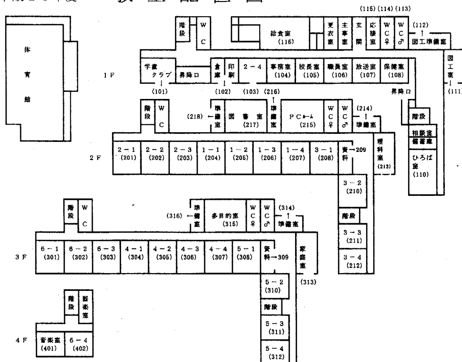
平成25年度 教室配置図
